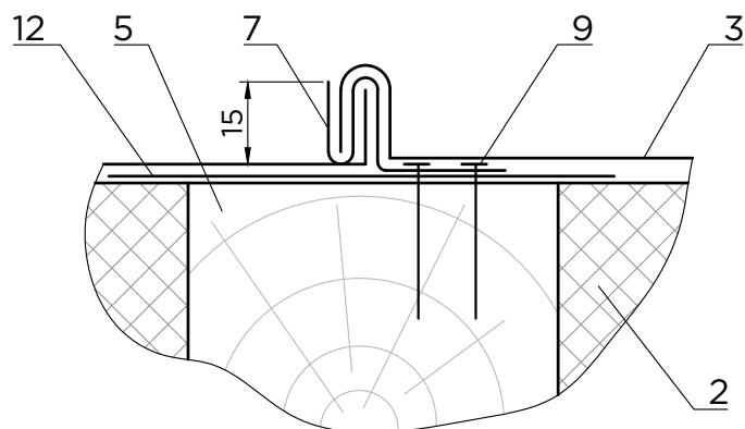
3 - 3
