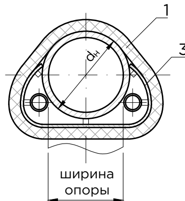
A - A с двумя спутниками
