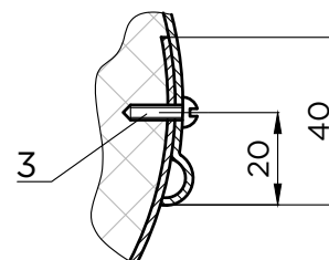
Д - Д
